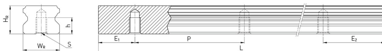
EGR_T profilsín méretei
